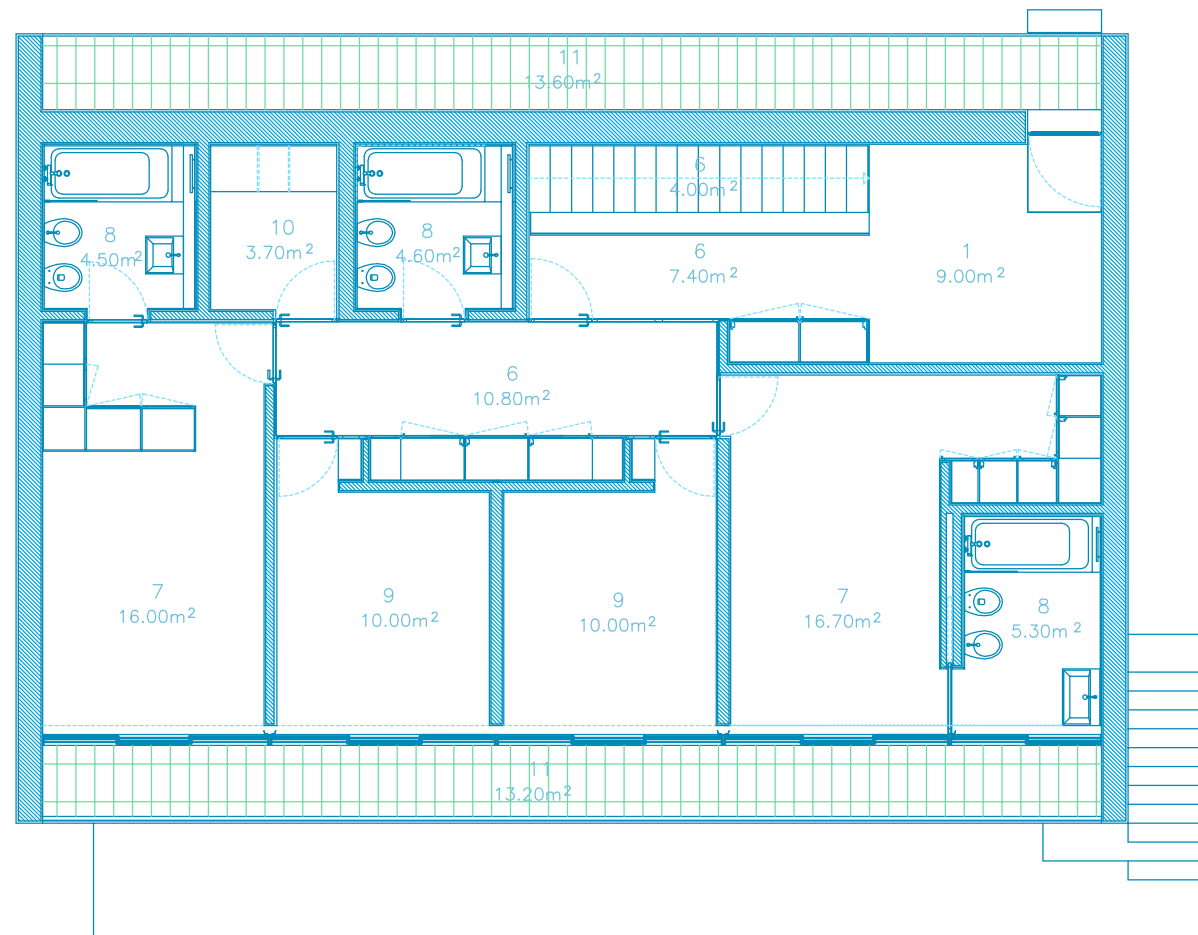
PLANTA PISO 0
