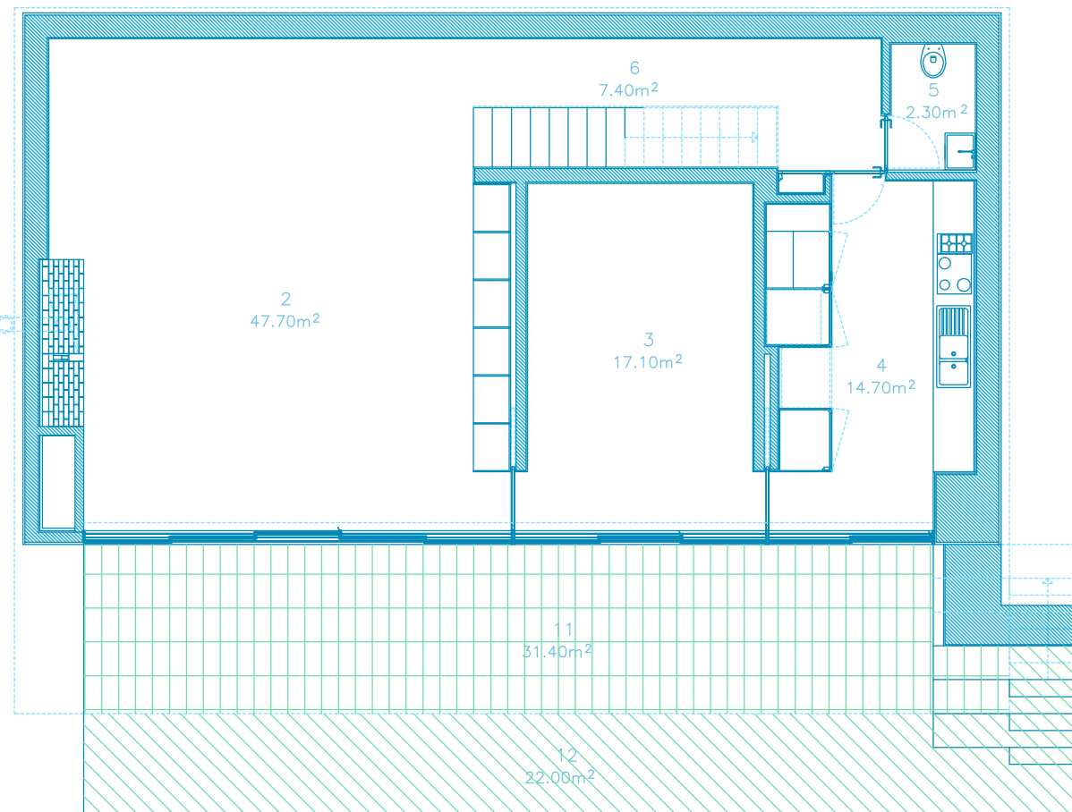
PLANTA PISO -1
